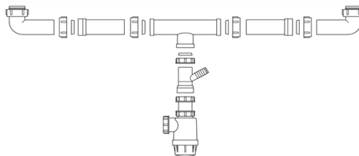
Sifón, Fitting y T para Lavavajilla
