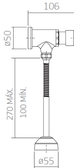
Dibujo Técnico
